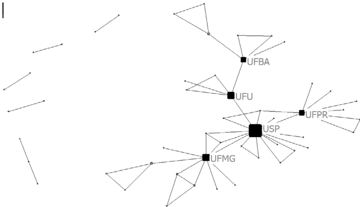
Figura 6: Rede social das IES – Centralidade de intermediação ( betweenness )
