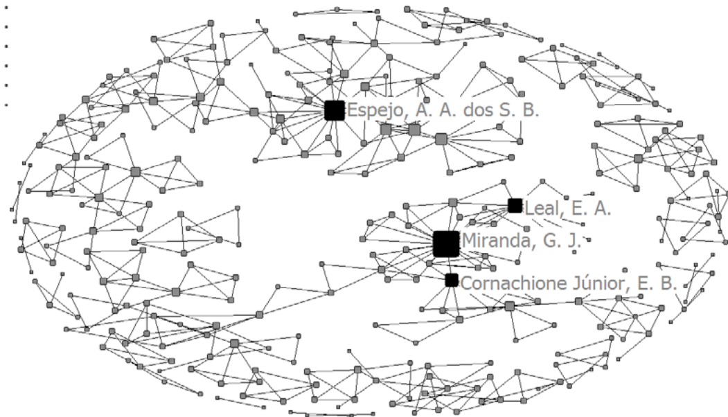
Figura 3: Redes de coautoria – Centralidade de grau ( degree )
