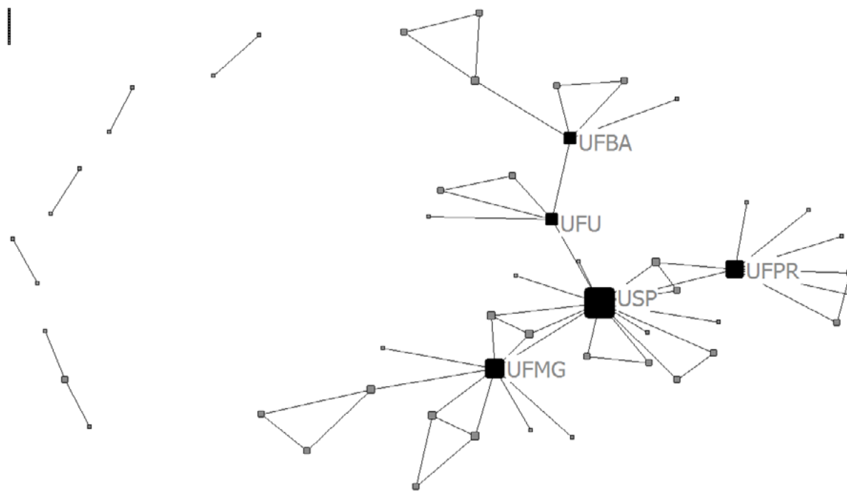
Figura 5: Rede Social das IES – Centralidade de grau ( degree )
