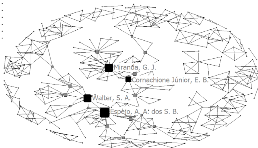
Figura 4: Redes de coautoria – Centralidade de intermediação ( betweenness )
